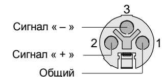
Распайка соединителя XLR (female)
